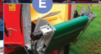
Przeñośniki wyładowcze W modelach wozów z pionowymi ślimakami wyposażonych w drzwi boczne dostępna jest opcja zamontowania hydraulicznych przeñośników wyładowczych umożliwiających podawanie do karmideł.
